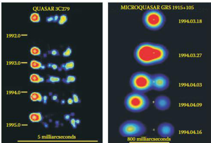
Obr. 6. Převzatý. Relativistické jety z kvasaru 3C279 (vlevo, aktivního galaktického jádra ) a mikrokvasaru GRS
