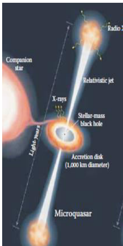
Obr. 8. Převzatá část. Binární systém. Vlevo je „hvězda společnice.“ Druhou částí systému (uprostřed obr.) je černá díra.
