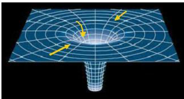
Obr. 10. Převzatý z internetu, doplněný o Susskindovu představu pádu bitů do černé díry (žluté šipky).
