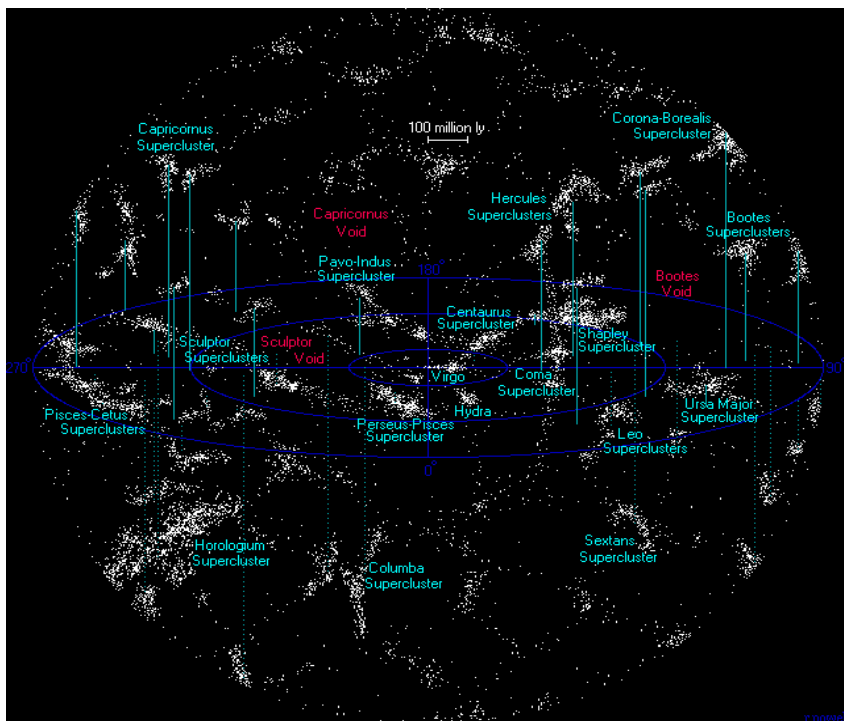
Obr. 3. Velkoměřítková struktura vesmíru.
