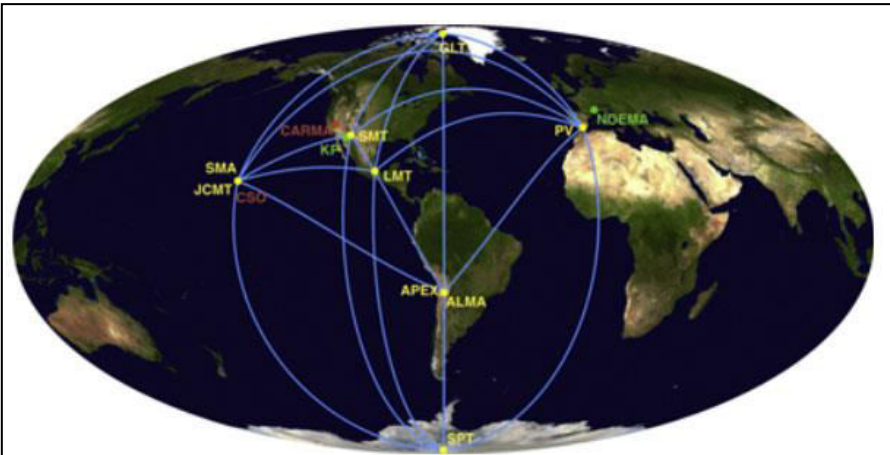
Obr. 17. Mapa stanic EHT. Stanice aktivní v r. 2017 a 2018 jsou ukázány spojovacími čarami a označeny žlutě, objednaná místa jsou označena zeleně, stará místa červeně.
