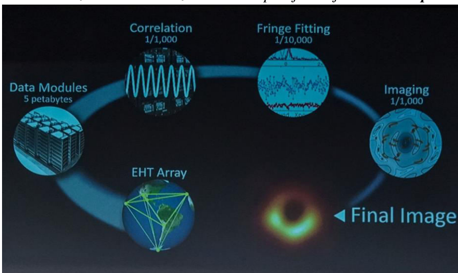
Obr. 15. Převzatý. Dlouhá cesta ke konečnému obrazu
