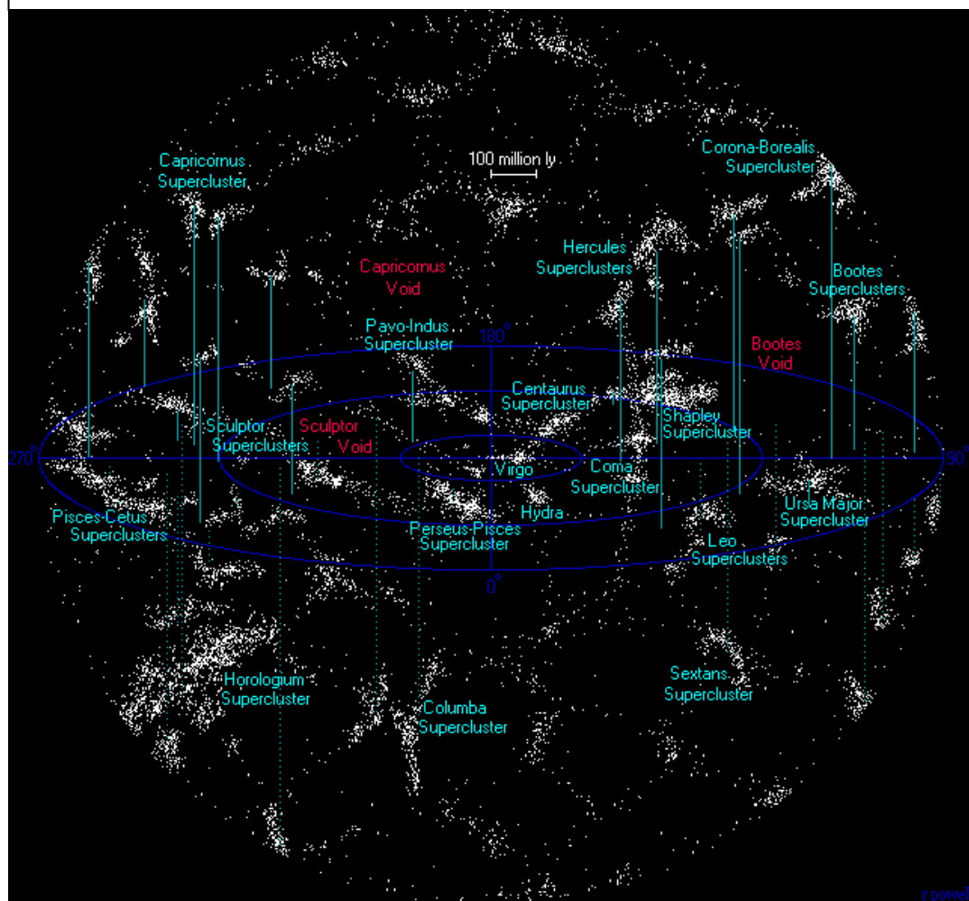
Obr. 7. Velkoměřítková struktura vesmíru. Převzato z: www.astro.pef.zcu.cz/objekty/obr/
