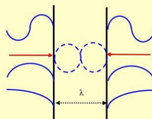
Obr.3. Vakuové síly přitlačují desky k sobě
