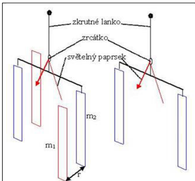
Obr. 4. Otcova torzní kyvadla. Vlevo: Původní uspořádání podobné Cavendishovu. Vpravo: Jen kyvadlo bez „pevných“ hmot m_1 .
