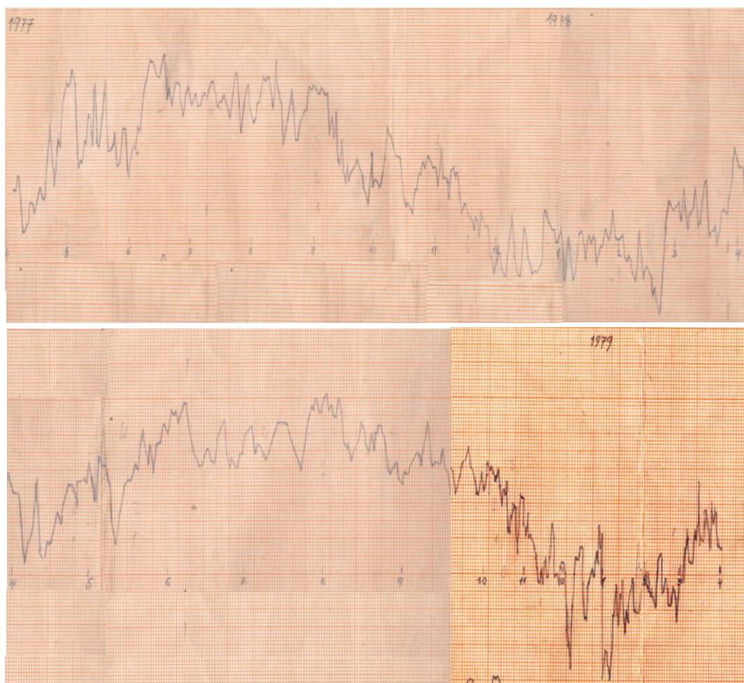
Obr. 3. Naskenovaná kopie originálního grafu, nakresleného mým otcem tužkou na milimetrový papír, odpovídající obr. 5. (dělanému bod po bodu z originálu ve wordové funkci „graf“). Nyní je vhodné použít zvětšení na monitoru.
