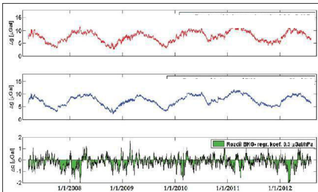
Obr. 8. Převzatý. „Nahoře: časová řada změn tíhového zrychlení na GO Pecný pro dvě metody zadávání atmosférické korekce: a) regresivní koeficient 0,3 \mu\text{Gal/hPa} , b) kombinace ATMACS a regresivního koeficientu. Dole: rozdíl mezi dvěma přístupy k výpočtu atmosférických korekcí.
