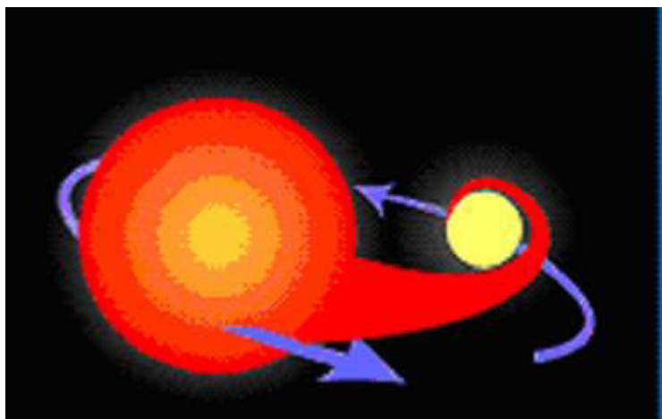
Obr. 17. Dvojhvězda. Z hvězdy obra na hvězdu trpaslíka: Těleso s menší hmotností přitahuje více ??
