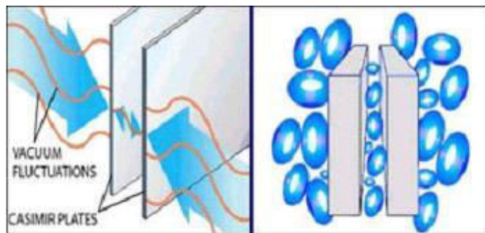
Obr. 21. Casimirův jev. X. Borg přebírá z internetu
