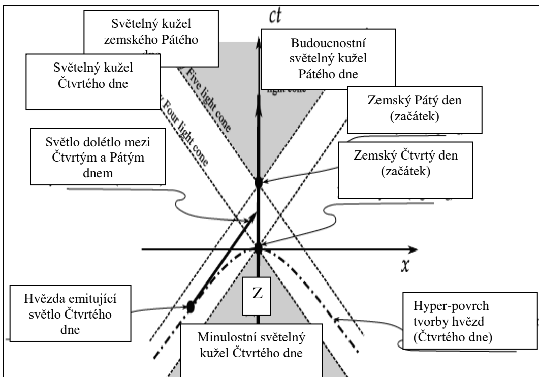
Obr. 4. Převzatý. Právě stvořená hvězda emituje světlo též den (4.) Je umístěna na hyperpovrch (hyperboloidu). To světlo letí až téměř k povrchu Země mimo (minulostní) světelný kužel, tzn. rychlostí větší než c . Přitom „souřadnice x představuje vzdálenost od Země, zatímco souřadnice ct představuje čas kalibrovaný rychlostí světla c .“
