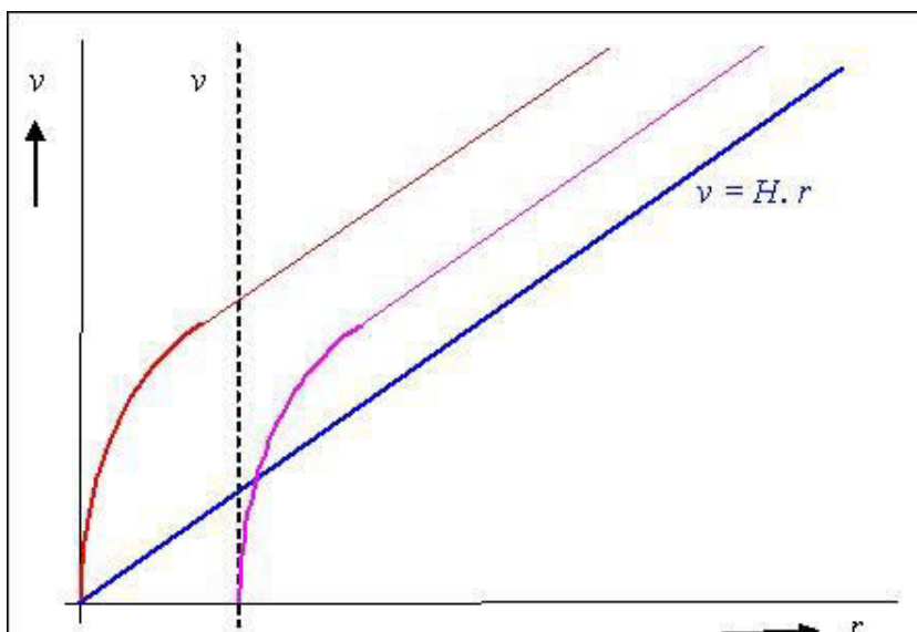
Obr. 16. Kde je počáteční bod údajného růstu rozpínání?
