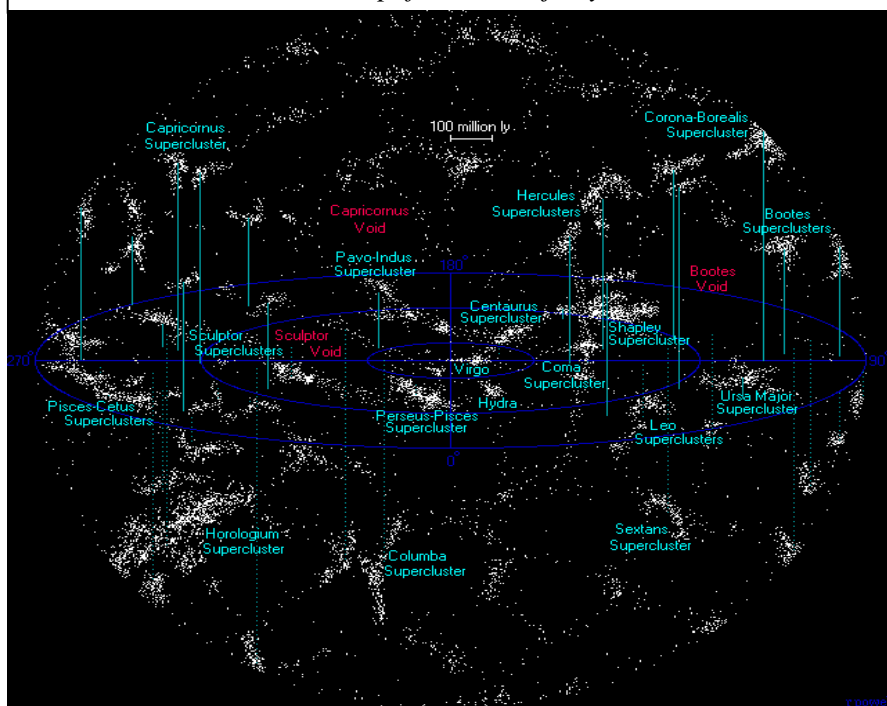
Obr. 11. Velkoměřítková struktura vesmíru. Převzato z: www.astro.pef.zcu.cz/objekty/obr/
