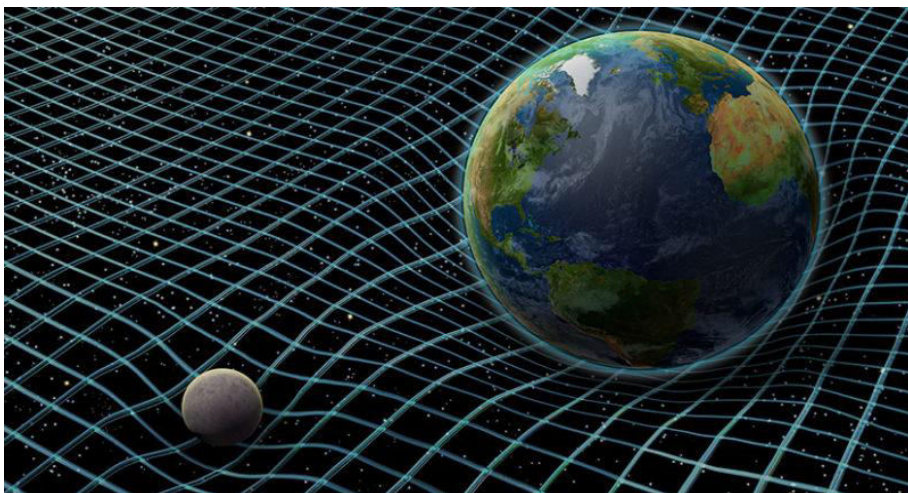
Obr. 4. Správný obr. Prostor je prohnutý jak pod Zemí, tak pod Měsícem. Měsíc v menším „důlku“ si vůbec nevšímá vzdálenější, i když větší prohlubně pod Zemí! Ty prohlubně jsou vzájemně nezávislé! Převzato z
