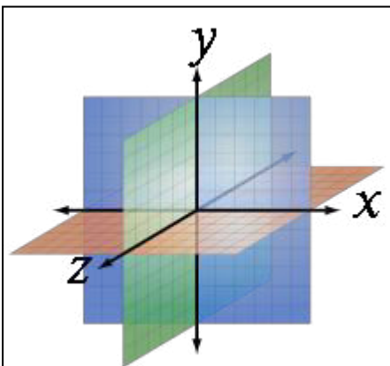
Obr. 2. 3D geometrický prostor. Převzato z
